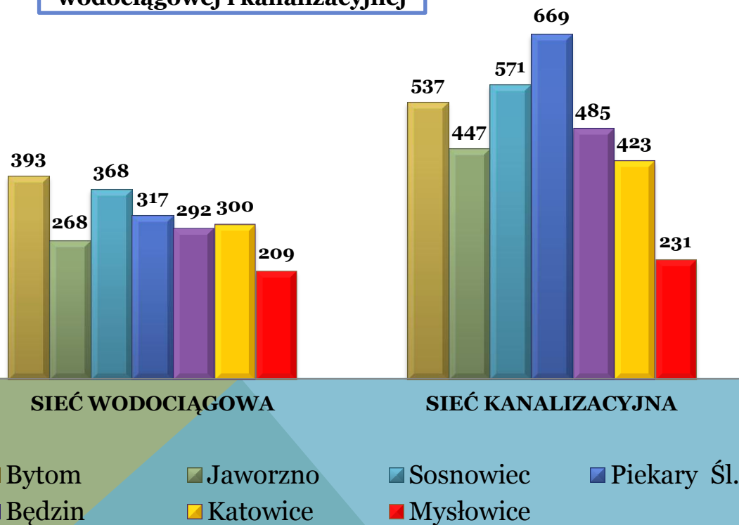
Ilość mieszkańców na 1 km sieci wodociągowej i kanalizacyjnej
